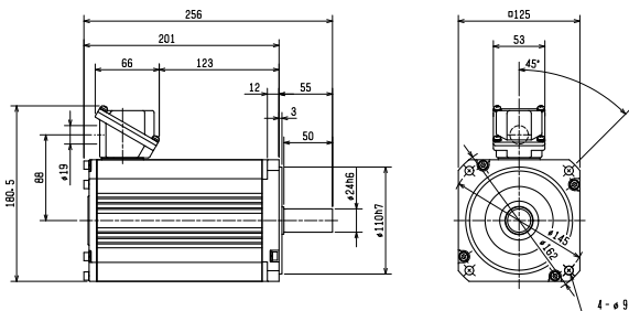
EM-AMF 3.7kW
