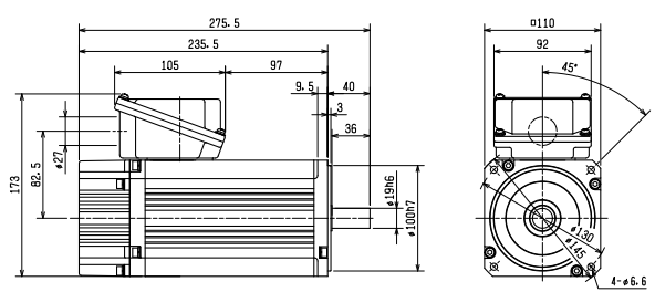
EM-AMFB 2.2kW
