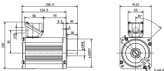
EM-AMF 1.5kW
