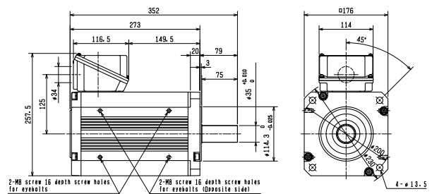
EM-AMF 5.5kW
