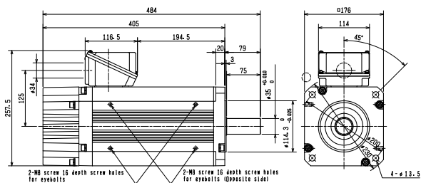
EM-AMFB 7.5kW
