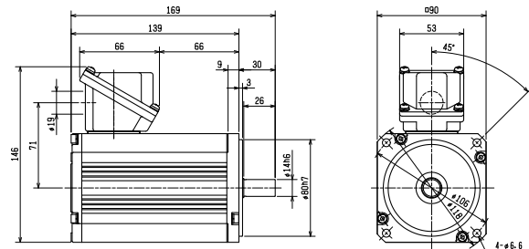
EM-AMF 0.75kW
