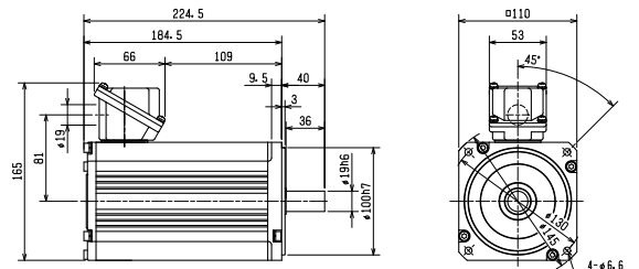
EM-AMF 2.2kW
